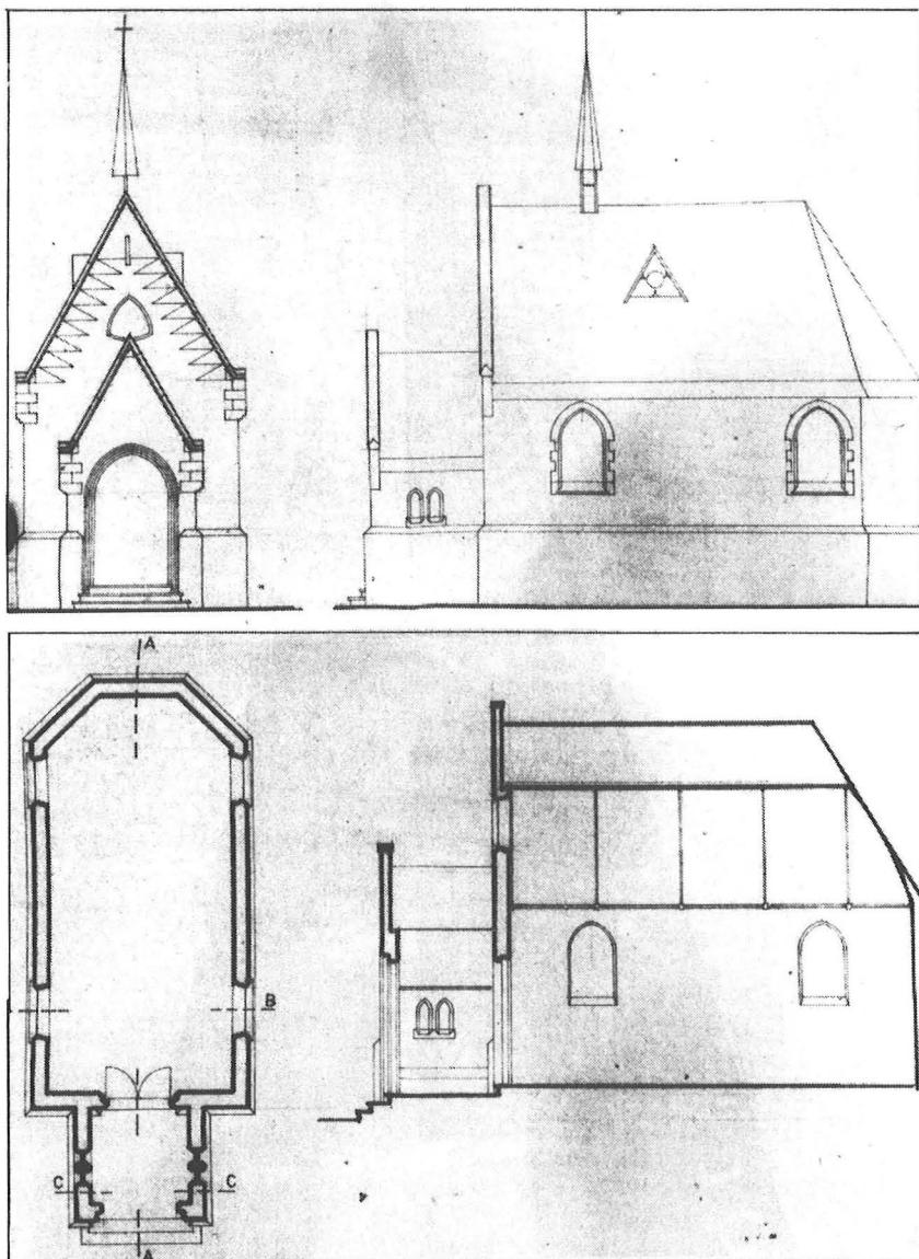
Grondplan en doorsnede A - B
